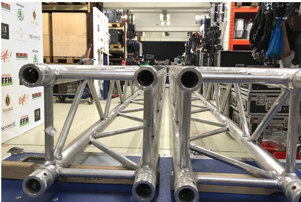
Abbildung 4: Vergleich einer 10 m Konusstrecke (links) gegenüber einer 10 m LITECRAFT TRUSS Klick made by RESBIG-Verbindungsstrecke
